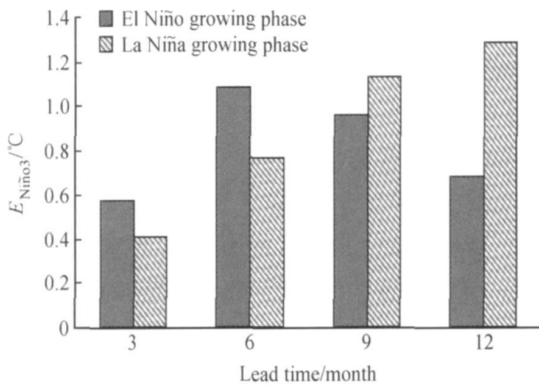
图 5 El Niño 事件和 La Niña 事件的 E_{Niño3} 随提前预报时间的变化。初始时刻为 El Niño (0) 1 月和 La Niña (0) 1 月 Fig 5 E_{Niño3} of the El Niño event and La Niña event, as a function of lead time. For start month El Niño (0) Jan and La Niña (0) Jan
