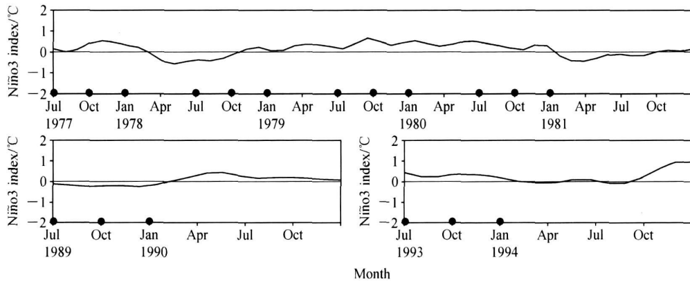
图 2 1972~ 1999 年正常年份的观测 Niño 3 指数。横坐标上的 “•” 表示预报的初始时刻
