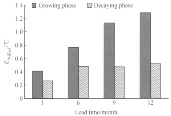
图 4 La Niña 事件的 E_{\text{Niño}3} 随提前预报时间的变化。初始时刻分别为 La Niña (0) 1 月和 La Niña (1) 1 月 Fig. 4 E_{\text{Niño}3} of the La Niña event, as a function of lead time. For start month La Niña (0) Jan and La Niña (1) Jan, respectively
