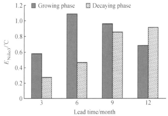
图 3 El Niño 事件的 E_{\text{Niño}3} 随提前预报时间的变化。初始时刻分别为 El Niño (0) 1 月和 El Niño (1) 1 月 Fig. 3 E_{\text{Niño}3} of the El Niño event, as a function of lead time. For start month El Niño (0) Jan and El Niño (1) Jan, respectively
