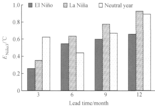
图8 同图7, 但不包括1997/1998年El Niño事件
