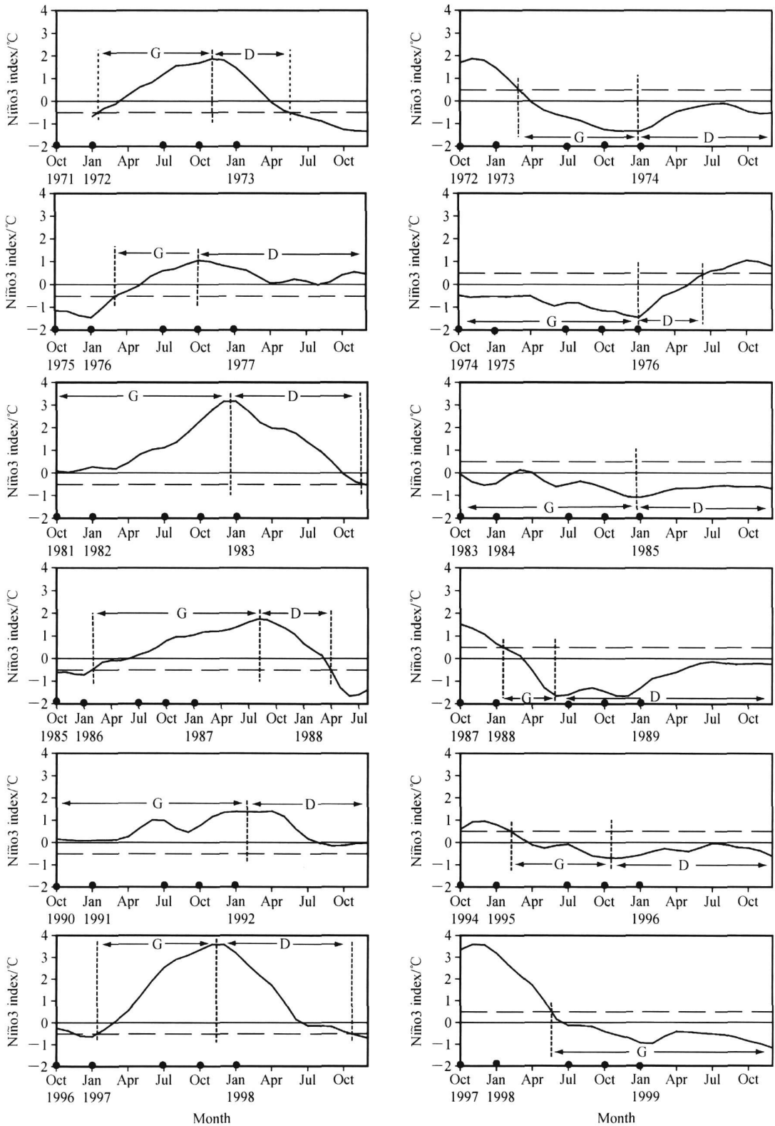
图1 1972~1999年6次El Niño事件(左列)和6次La Niña事件(右列)的观测Niño3指数。G表示生长期, D表示衰减期, 横坐标上的“•”表示预报的初始时刻
