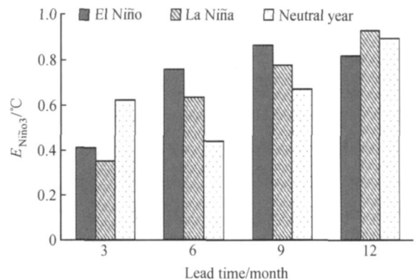
图 7 1972~1999 年 El Niño 事件、La Niña 事件和正常年份的 E_{Niño3} 随提前预报时间的变化。初始时刻为 1 月 Fig 7 E_{Niño3} of the El Niño event, La Niña event and neutral year during 1972-1999, as a function of lead time. For start month Jan
