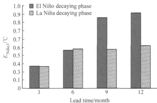
图 6 El Niño 事件和 La Niña 事件的 E_{Niño3} 随提前预报时间的变化。初始时刻为 El Niño (1) 1 月和 La Niña (1) 1 月 Fig 6 E_{Niño3} of the El Niño event and La Niña event, as a function of lead time. For start month El Niño (1) Jan and La Niña (1) Jan
