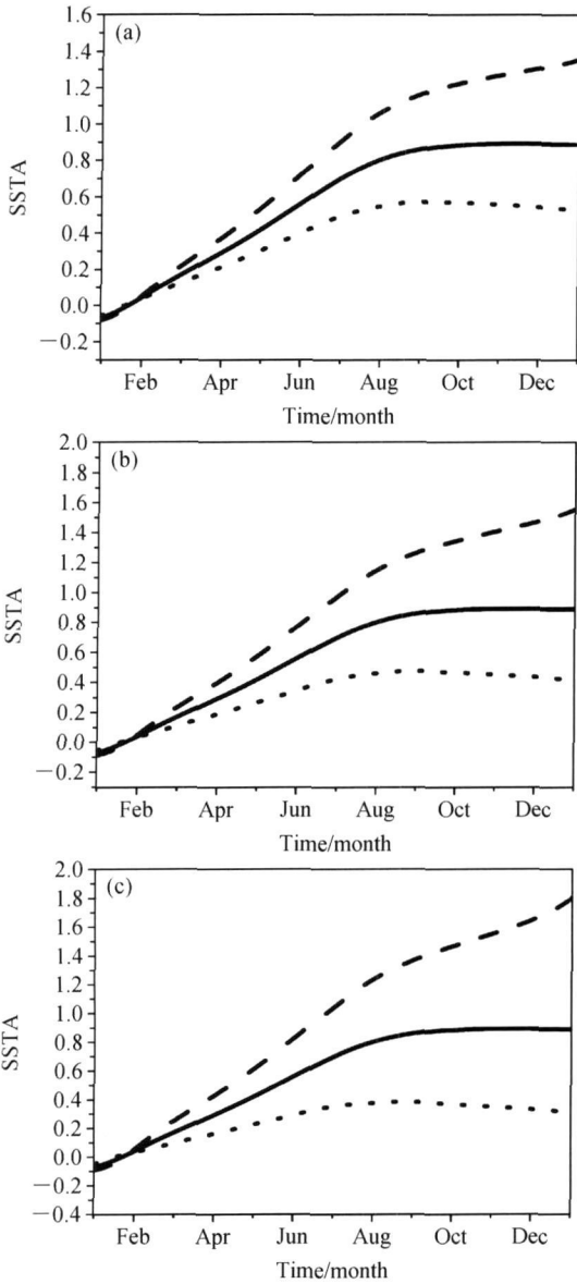
图5 由CNOP-P (虚线) 以及局部 CNOP-P (点线) 所表征的赤道高频纬向风强迫影响下的 El Niño 事件及 El Niño-1 (实线)。参数约束分别为: (a) \sigma_1=0.3, \sigma_2=0.3, \sigma_3=0.6 ; (b) \sigma_1=0.4, \sigma_2, \sigma_3 同 (a); (c) \sigma_1=0.5, \sigma_2, \sigma_3 同 (a)。
