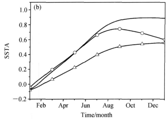
图 9 当参数约束为 \sigma_1=0.5 , \sigma_2=0.3 , \sigma_3=0.6 时, 由 (a) CNOP-P 和 (b) 局部 CNOP-P 所表征的赤道高频纬向风强迫被带入 Model-1 (圆圈线) 以及 Model-2 (三角线) 得到的 El Niño 事件。实线代表 El Niño-1。
