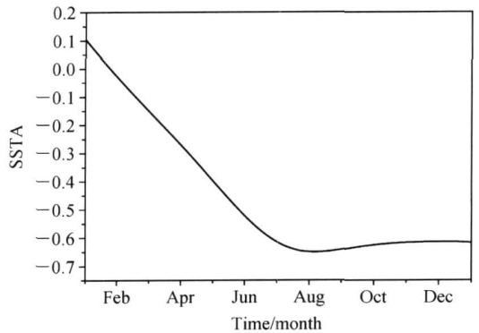
图 2 La Niña-1: WF96 模式中的一次 La Niña 事件, 其初始距平为 (0.1073, -0.1219)
