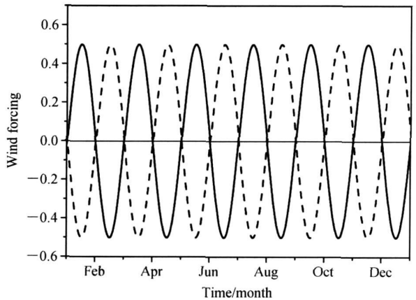
图 4 当参数约束为 \sigma_1=0.5, \sigma_2=3, \sigma=0.6 时, La Niña-1 情形下由 CNOP-P (实线) 以及局部 CNOP-P (虚线) 所表征的赤道高频纬向风强迫
