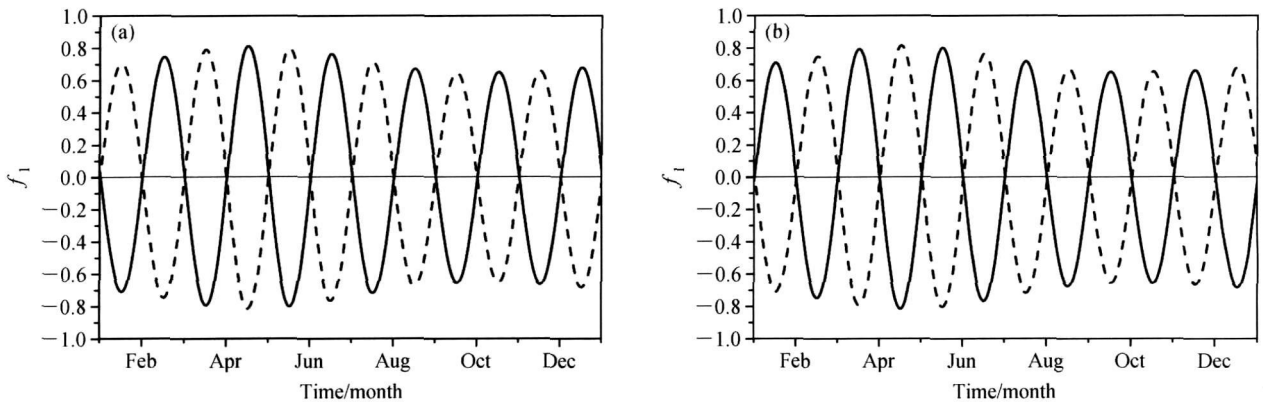
图 7 当参数约束为 \sigma_1=0.5, \sigma_2=0.3, \sigma_3=0.6 时, (a) El Niño-1 和 (b) La Niña-1 情形下由 CNOP-P (实线) 以及局部 CNOP-P (虚线) 所表征的强迫项 f_1
