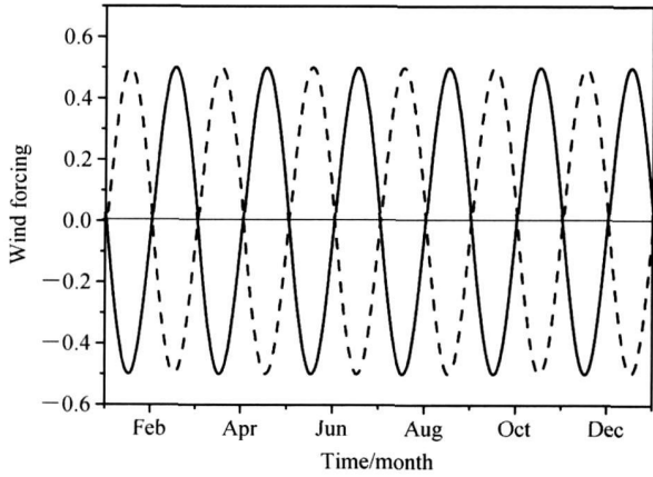
图 3 当参数约束为 \sigma_1=0.5, \sigma_2=3, \sigma=0.6 时, El Niño-1 情形下由 CNOP-P (实线) 以及局部 CNOP-P (虚线) 所表征的赤道高频纬向风强迫
