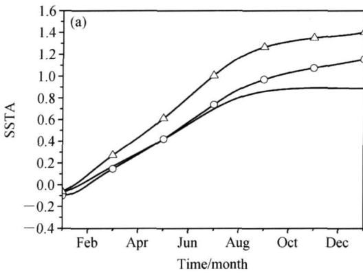
图 9 当参数约束为 \sigma_1=0.5 , \sigma_2=0.3 , \sigma_3=0.6 时, 由 (a) CNOP-P 和 (b) 局部 CNOP-P 所表征的赤道高频纬向风强迫被带入 Model-1 (圆圈线) 以及 Model-2 (三角线) 得到的 El Niño 事件。实线代表 El Niño-1。
