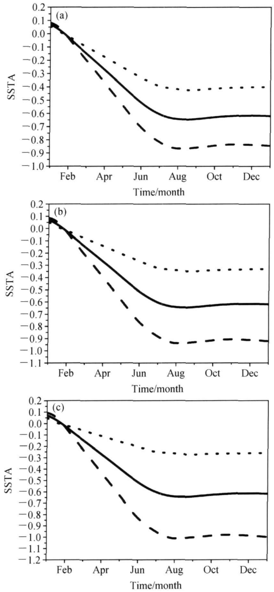
图6 由CNOP-P (虚线) 以及局部 CNOP-P (点线) 所表征的赤道高频纬向风强迫影响下的 La Niña 事件及 La Niña-1 (实线)。参数约束分别为: (a) \sigma_1=0.3, \sigma_2=0.3, \sigma_3=0.6 ; (b) \sigma_1=0.4, \sigma_2, \sigma_3 同 (a); (c) \sigma_1=0.5, \sigma_2, \sigma_3 同 (a)。
