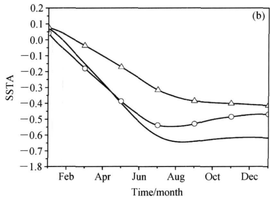
图 10 当参数约束为 \sigma_1=0.5 , \sigma_2=0.3 , \sigma_3=0.6 , 由 (a) CNOP-P 和 (b) 局部 CNOP-P 所表征的赤道高频纬向风强迫被带入 Model-1 (圆圈线) 以及 Model-2 (三角线) 得到的 La Niña 事件, 实线代表 La Niña-1
