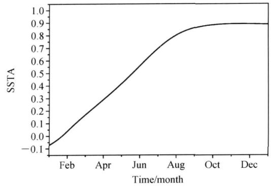
图 1 El Niño-1: WF96 模式中的一次 El Niño 事件, 其初始距平为 (-0.1102, 0.1423)
