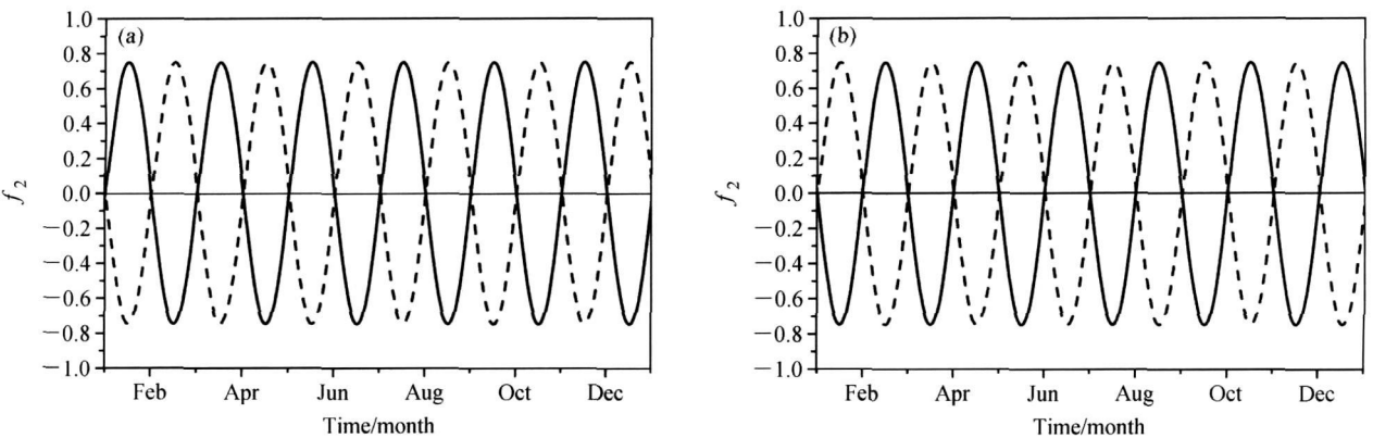
图 8 当参数约束为 \sigma_1=0.5, \sigma_2=0.3, \sigma_3=0.6 时, (a) El Niño-1 和 (b) La Niña-1 情形下由 CNOP-P (实线) 以及局部 CNOP-P (虚线) 所表征的强迫项 f_2
